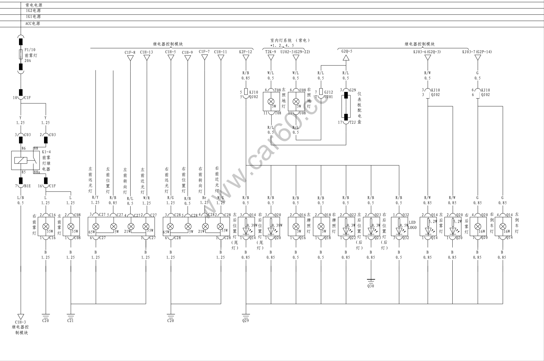
室外灯系统（大灯、位置灯、雾灯、牌照灯、倒车灯、LED LOGO）控制系统
